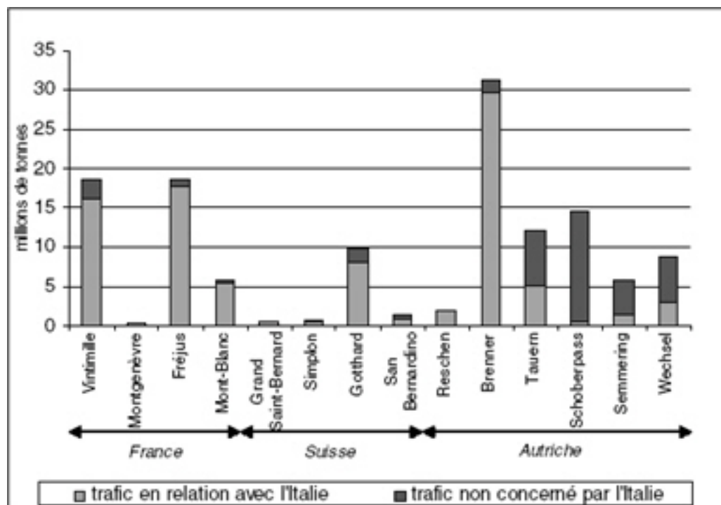
Fig. 55 – Trafic transalpin émis ou reçu par l'Italie (2004)
