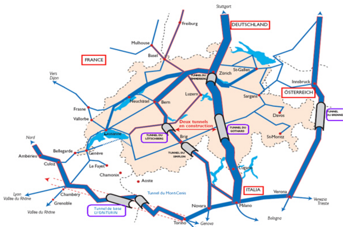
Fig. 20 – Les projets ferroviaires alpins
