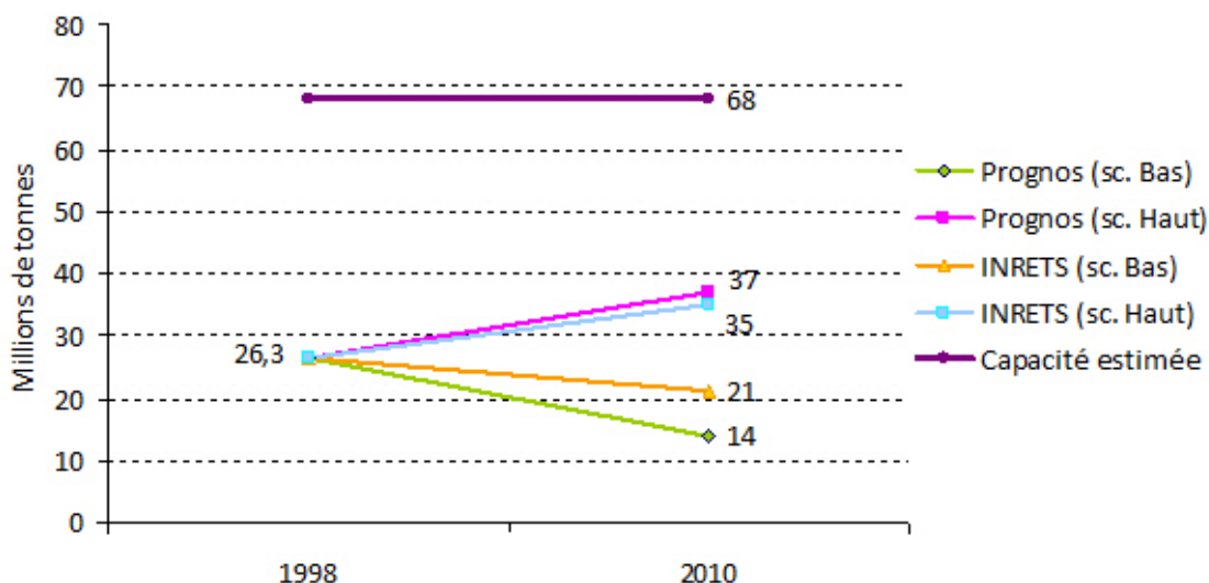
Fig. 29 – Les prévisions pour 2010 des flux aux passages routiers nord alpins français
