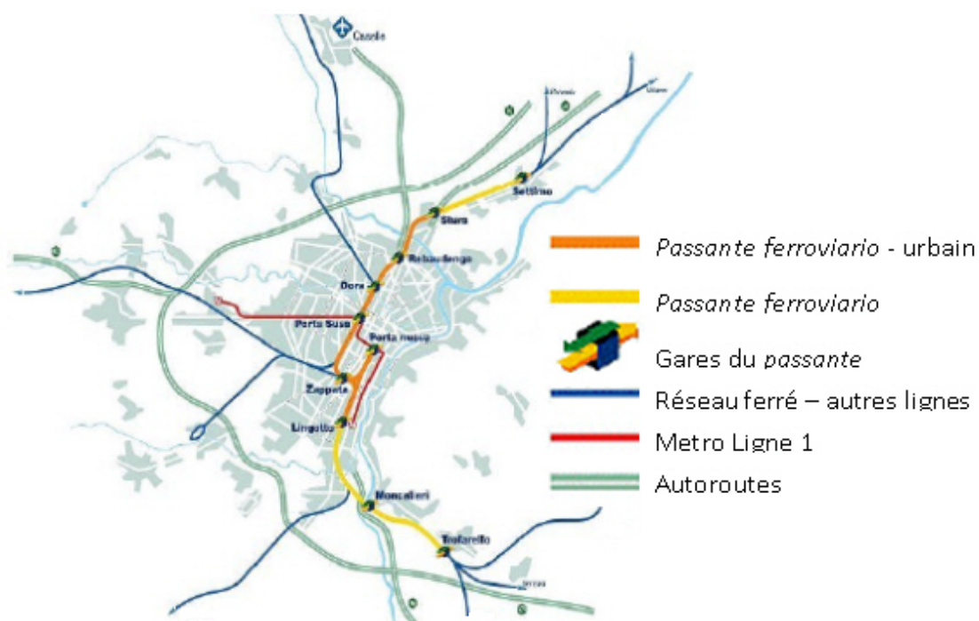
Fig. 38 - Passante ferroviario de Turin
