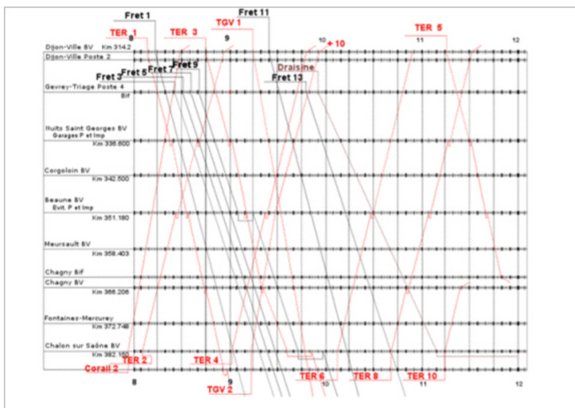
Fig. 5 – Graphique de circulation ferroviaire (fictif)
