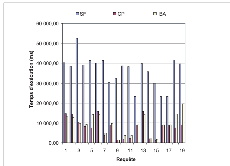
FIG. 6.4 – Temps d'exécution de la charge (configuration 2)
