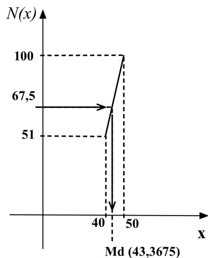
Figura 17 – Solução gráfica com determinação da mediana para os dados da tabela
