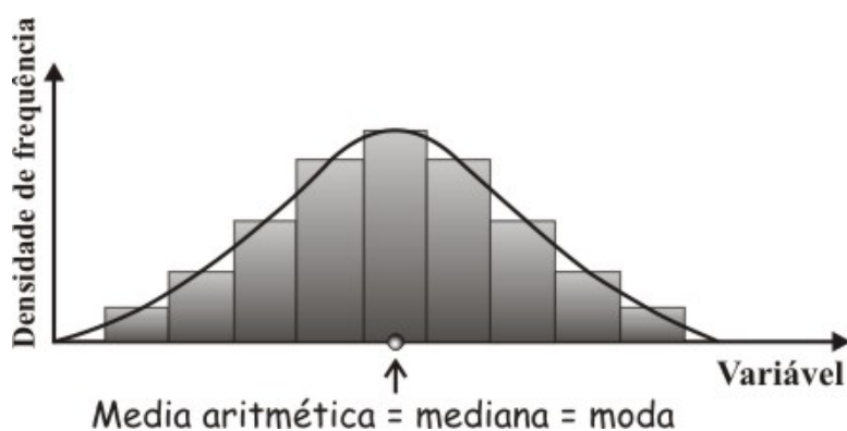
Gráfico 13 – A moda, mediana e média em uma distribuição simétrica dos dados.
