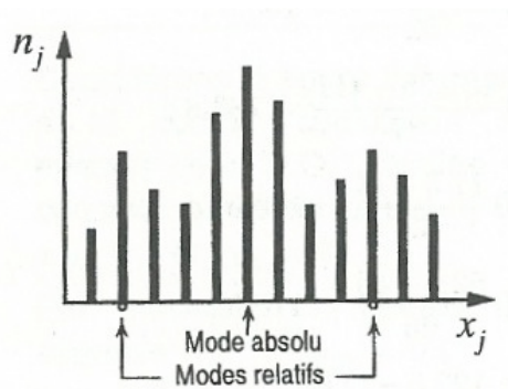
Gráfico 11 – Moda absoluta e relativa segundo Dehon, Droesbeke, Vermandele (2008)
