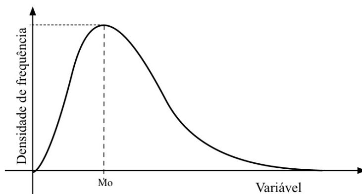
Gráfico 12 – Moda para dados contínuos.
