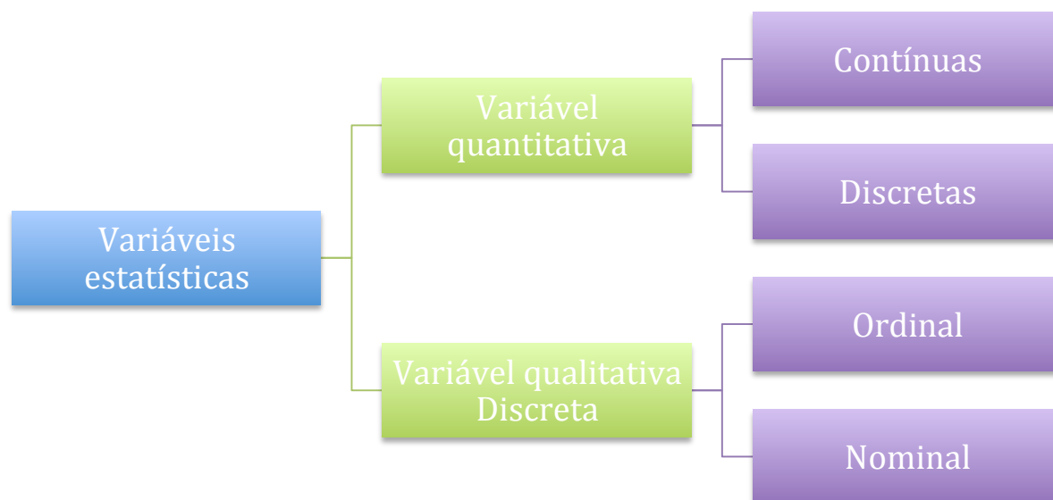
Figura 18 – Classificação das variáveis estatísticas segundo Régnier (2011a).
