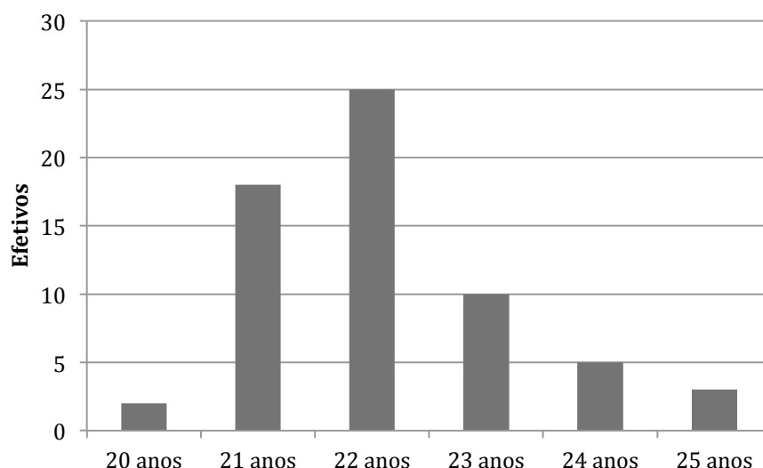
Gráfico 4 – Idade dos empregados de uma empresa A.
