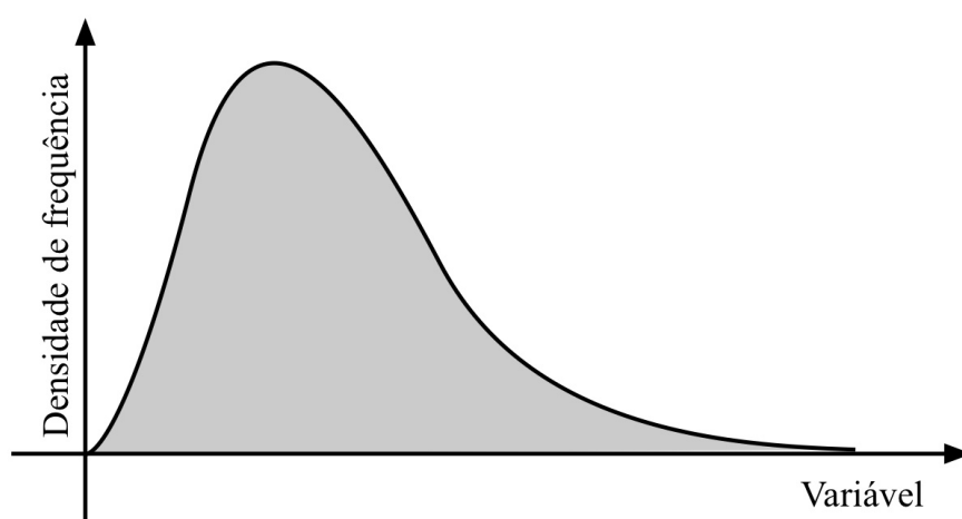
Figura 6 – Histograma de uma variável contínua.
