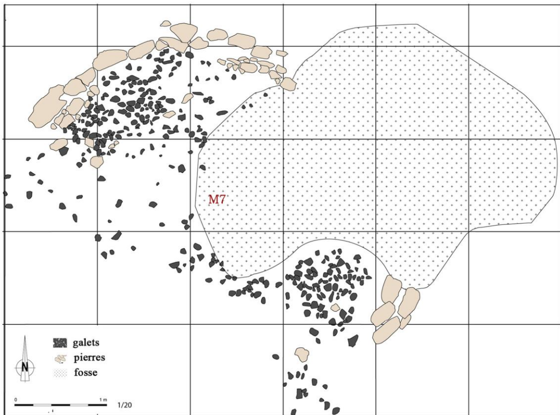
Fig. 19 – Photo et plan de la construction M7.
