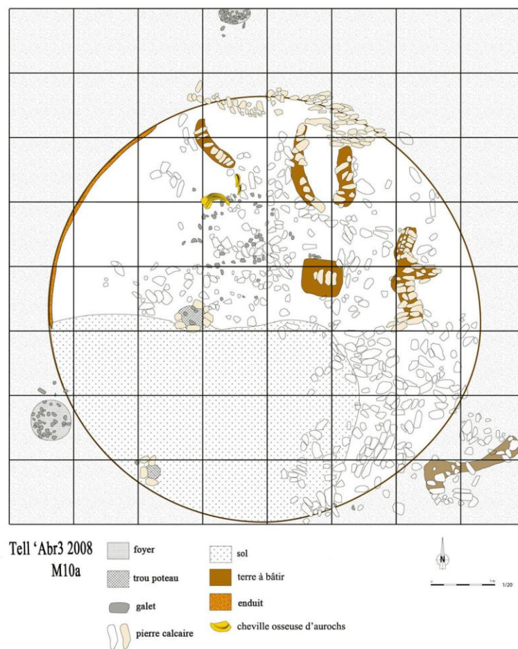
Fig. 26 – Photo et plan du bâtiment M10a.
