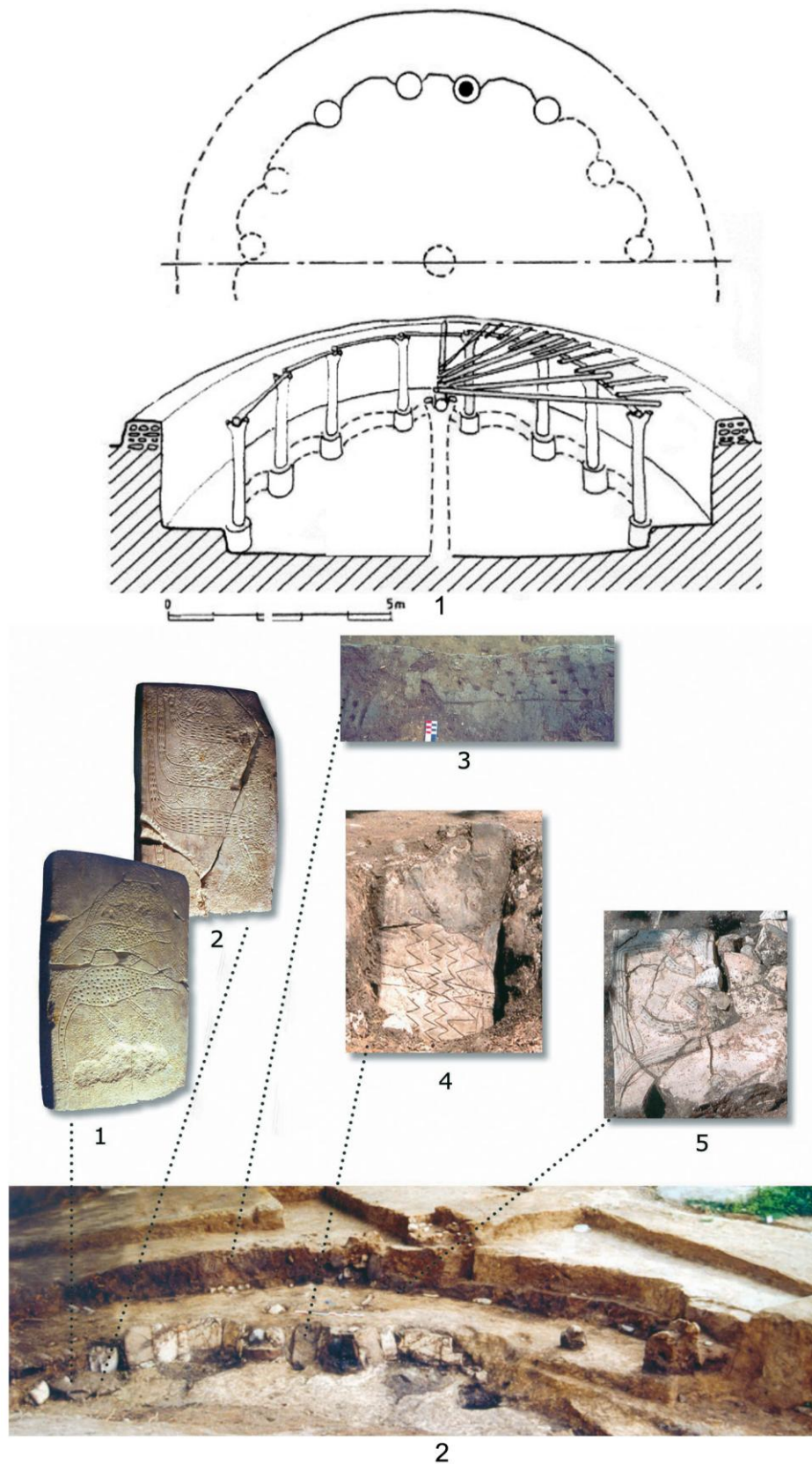
Fig. 112 – Bâtiment B2. 1 : reconstitution du bâtiment (dessin G. Deraprahamian) ; 2 : position des dalles décorées au front de la plateforme du bâtiment.
