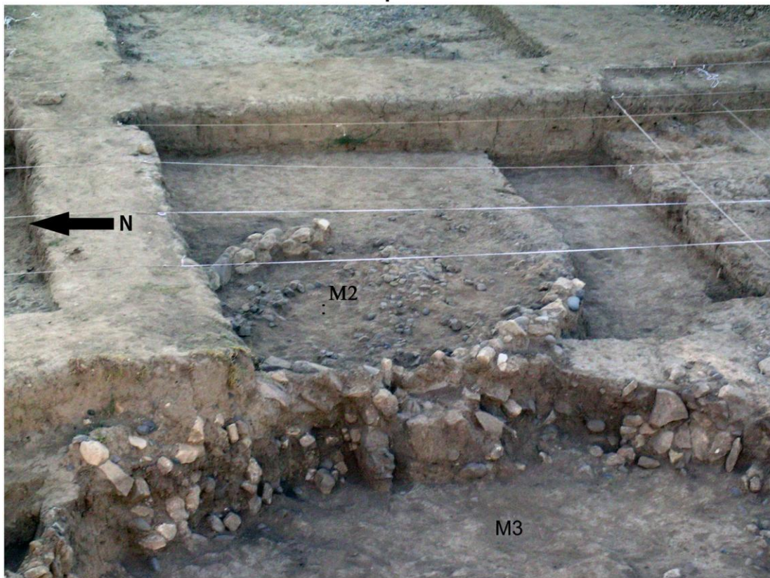
Fig. 98 – Construction M2. 1 : plan ; 2 : superposition d'une partie Ouest du mur de M2 sur le mur de soutènement de M3.
