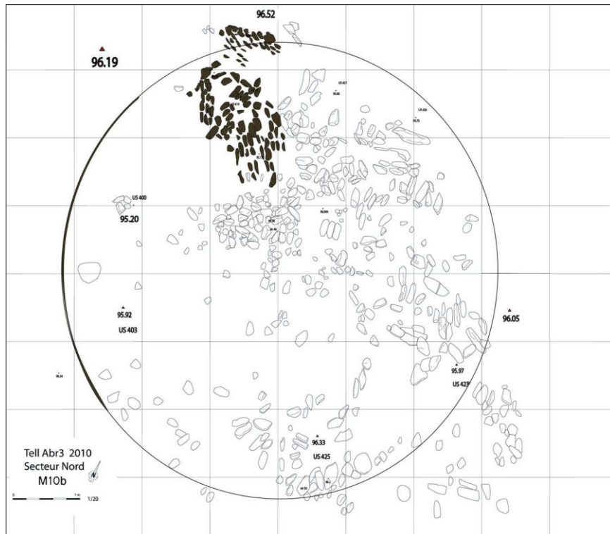
Fig. 37 – Plan de la destruction (A) du bâtiment M10b. Un mur est trouvé intact et effondré (en noir).
