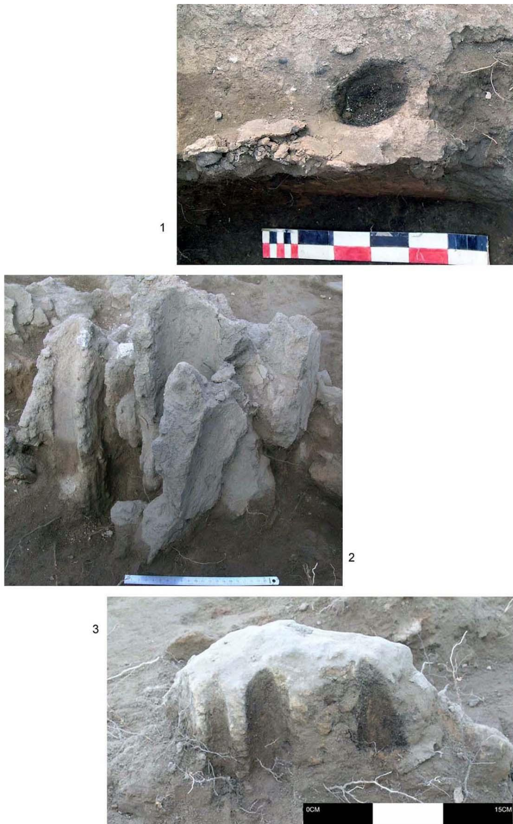
Fig. 64 – Bâtiment M1a. Poteaux et charpentes en bois. 1 et 3 : négatifs de poteaux sur la terre à bâtir enduite de la paroi du bâtiment; 2 : négatifs de charpentes sur la terre à bâtir du toit.
